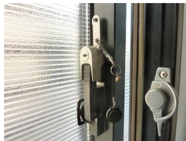
図. 引き違い戸に取り付けたもの 二重サッシの外側のクレセント錠に補強金具をつけてみました。
